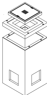
Topfschacht 100/100/200
