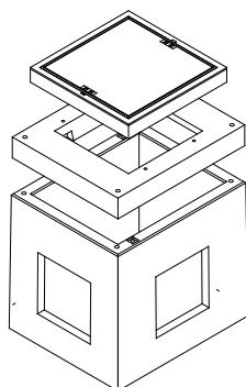
Topfschacht 100/80/100
