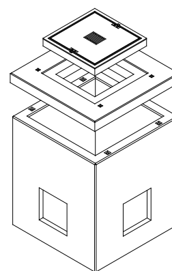
Topfschacht 120/120/150
