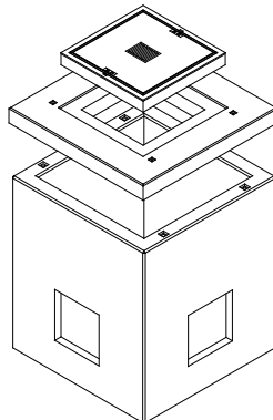
Topfschacht 120/120/100
