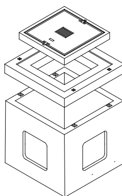
Topfschacht 100/100/100
