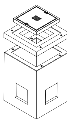
Topfschacht 120/120/150
