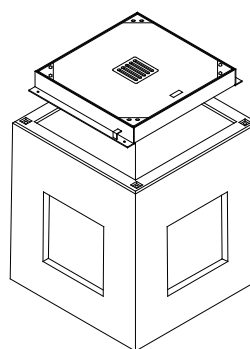
Topfschacht 80/80
