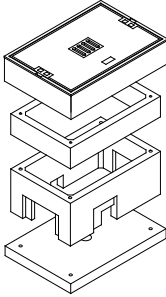
Abzweigkasten 65/40 Typ V Klasse B 125 + D 400
