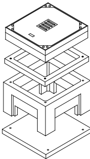
Kabeleinführungsplatten aus PE- HD
