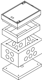
Abzweigkasten 65/60 Typ 2002 EP Klasse B 125 + D 400
