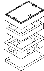
Abzweigkasten 65/40 Typ III Klasse B 125 + D 400
