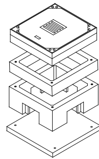
Abzweigkasten 65/60 Typ I / II Klasse B 125 + D 400
