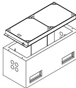
P-Schacht VI-A - 120/40/60 cm i.L. (als Aufbauschacht)
