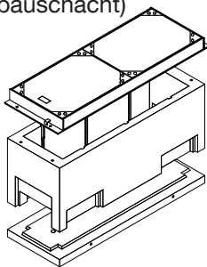
P-Schacht IV-A - 160/50/70 cm i.L. (als Aufbauschacht)
