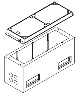
P-Schacht V-A - 174/68 cm i.L. (als Aufbauschacht, längsgeteilt)
