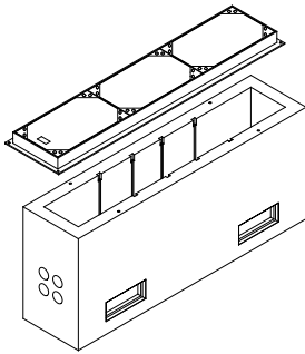
P-Schacht II-A - 160/40/70 cm i.L. (als Aufbauschacht)
