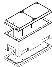
P-Schacht V-A - 174/68 cm i.L. (als Aufbauschacht, längsgeteilt)
