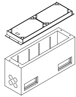
P-Schacht IV - 160/50/70 cm i.L.
