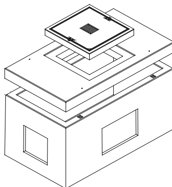
Topfschacht 200/100/100
