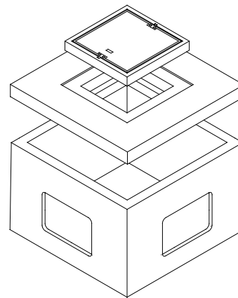
Topfschacht 150/150/100
