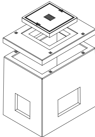
Topfschacht 150/100/150
