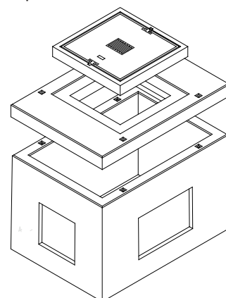
Topfschacht 200/150/100
