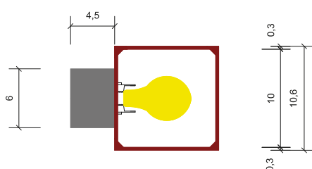
Draufsicht
